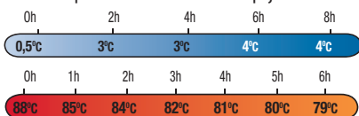
Rozkład temperatur w termosie do napojów XB:
